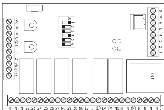
Fig. 10 Styrekort kryssaggregat
